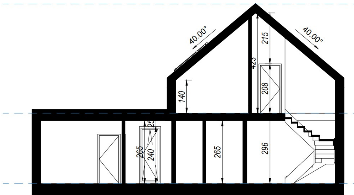
/ przekrój /
