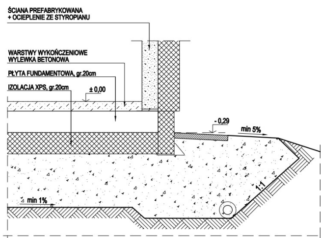
/ detal ciepłej płyty /
