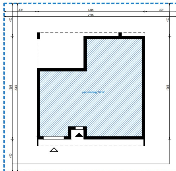
/ przykładowe usytuowanie budynku na działce 5a /
