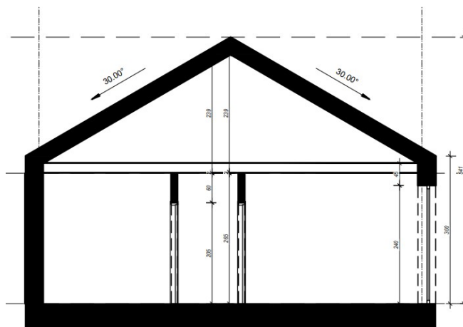
/ przekrój /
